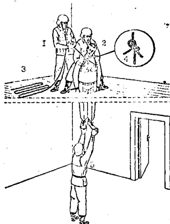
Спускание человека с помощью нагрудной перевязи.
